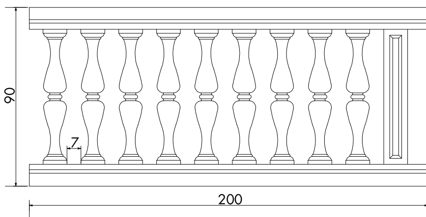
COMPOSIZIONE BALAUSTRADA
