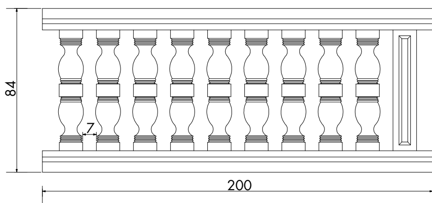
COMPOSIZIONE BALAUSTRATA
