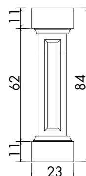
PILASTRINO
