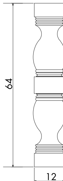
BALAUSTRINO 14/B Dim. cm. 12 x 12 x 64 h.
