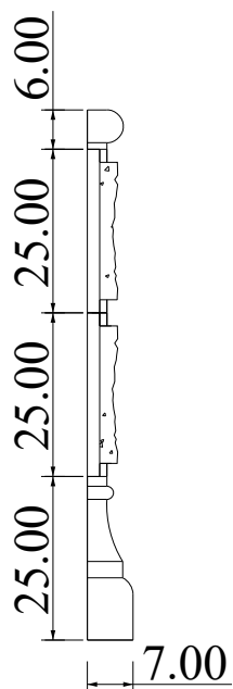
Sezione
